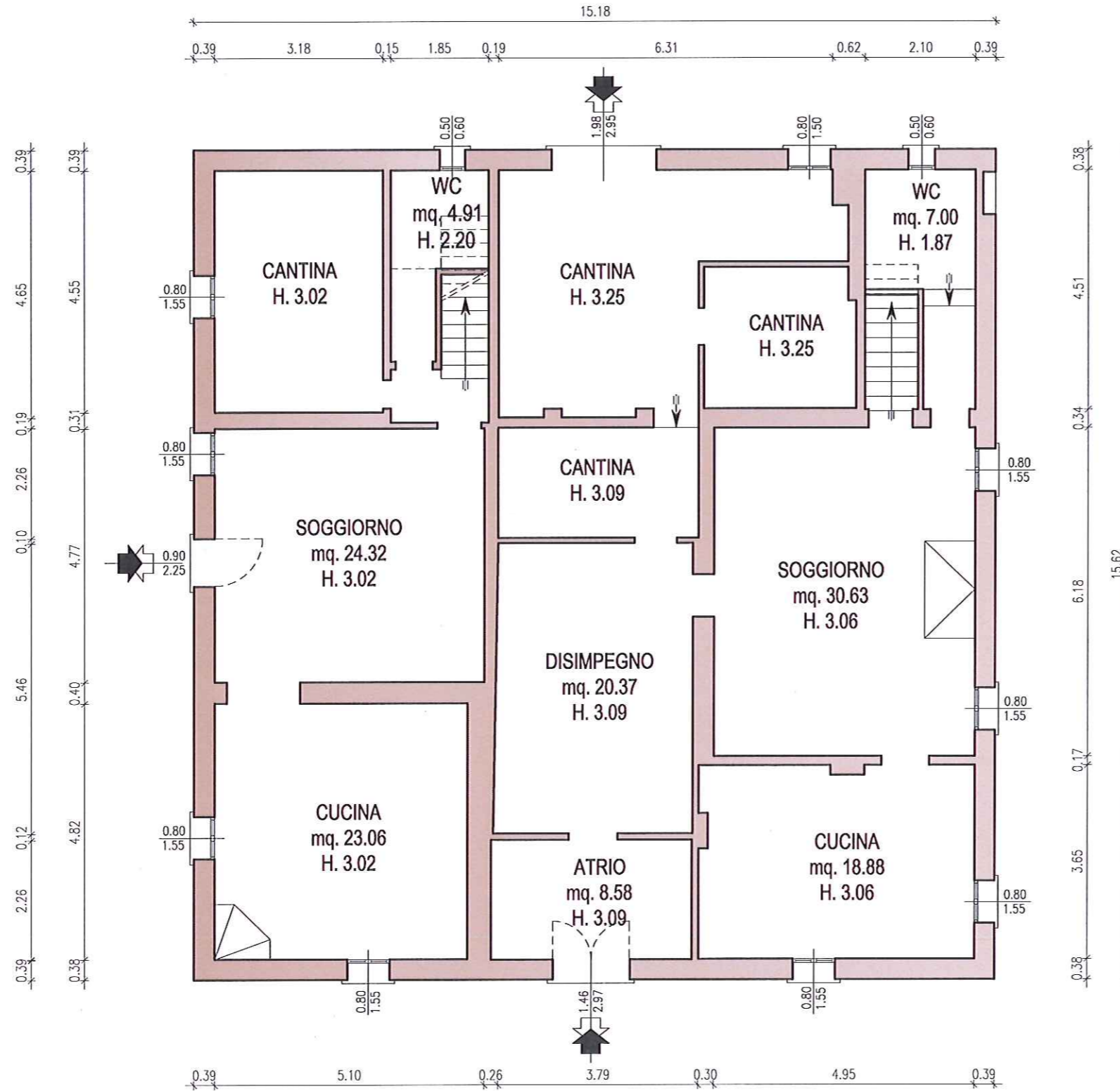
PIANO TERRA h. 3.09
