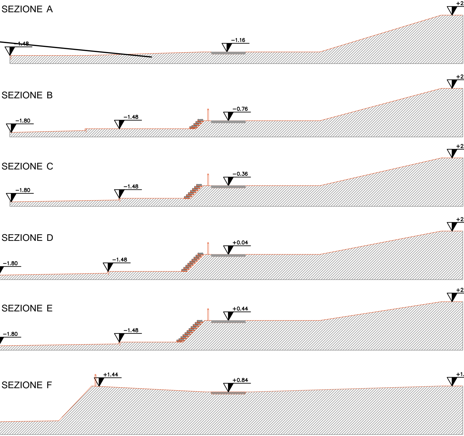
SEZIONI SU PISTA CICLABILE scala 1:200
