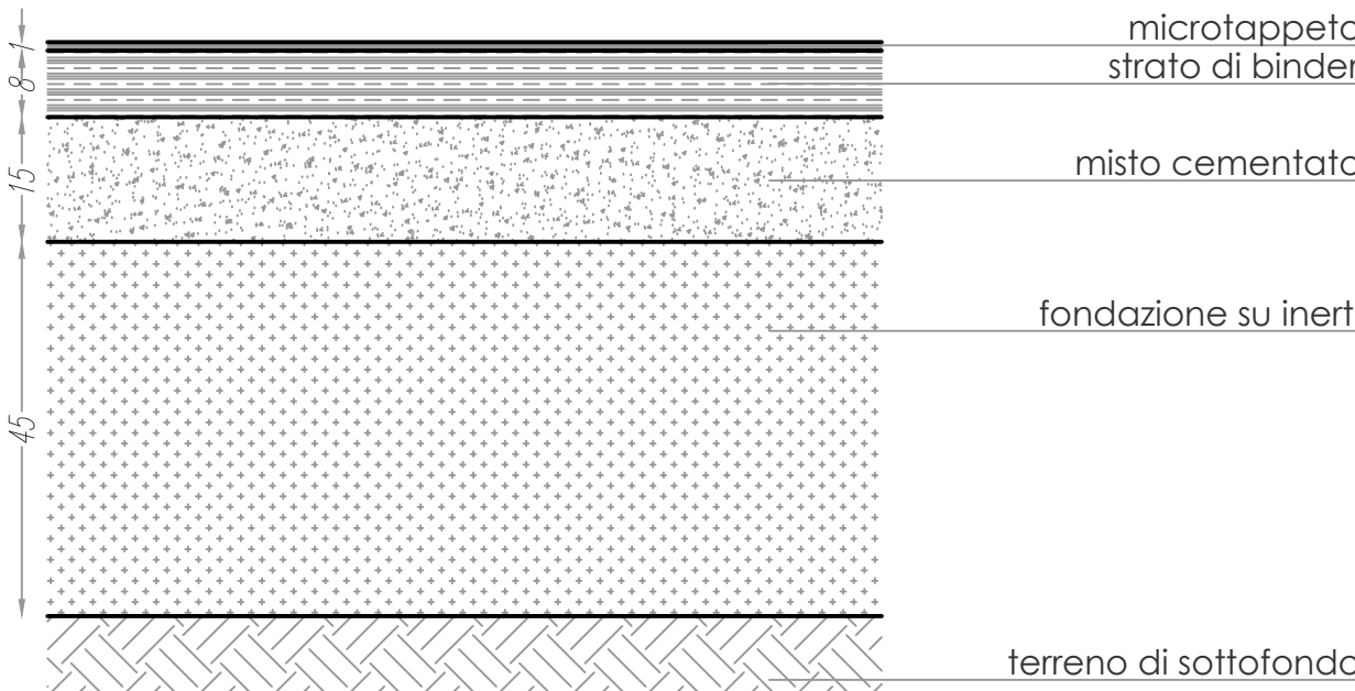
SCHEMA STRATIGRAFIA STRADALE TIPO
